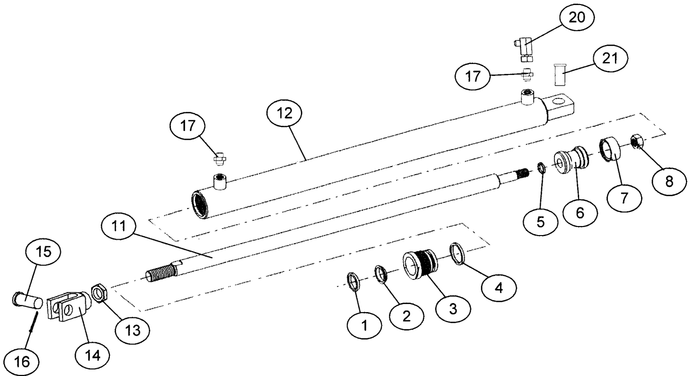
DE506014 - HYD. PISTON 50 X 25 X 550
